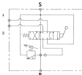
1 leva/lever
